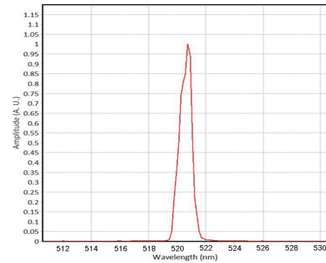
520nm激光光谱图
