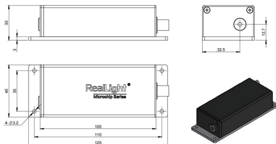
激光头尺寸图 (侧出光)
