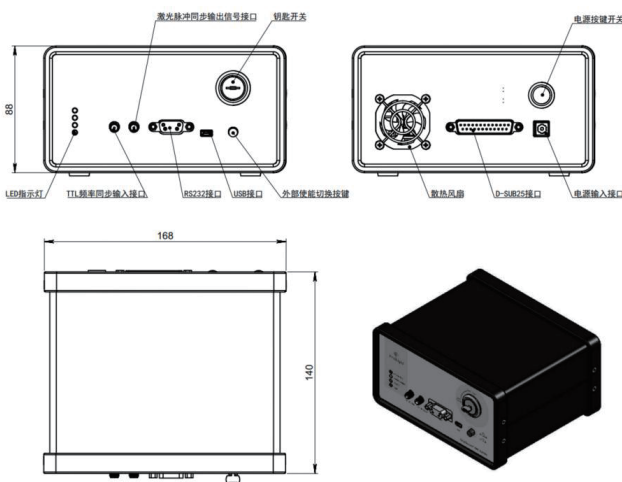
驱动电源尺寸图
