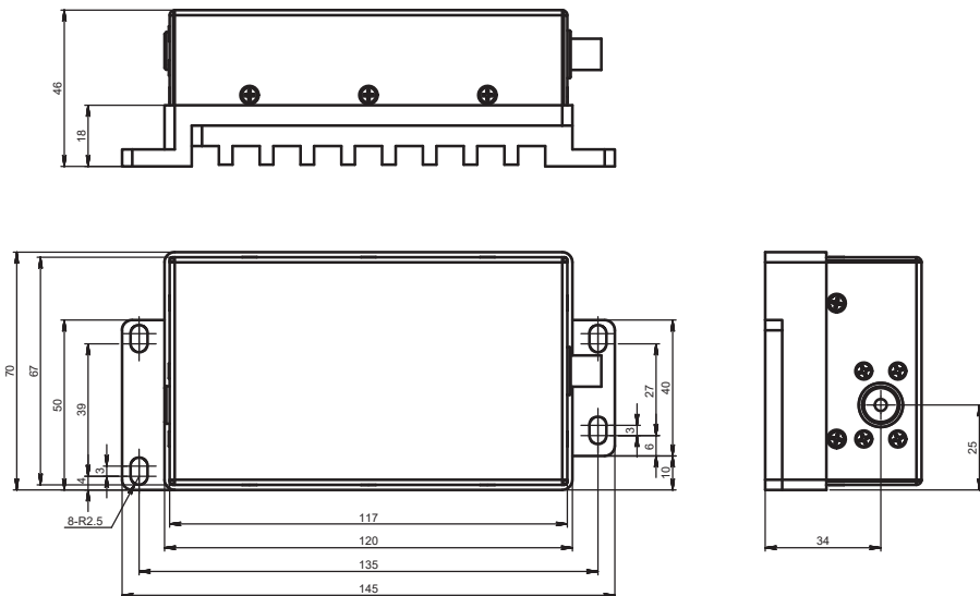
双脉宽激光头尺寸图
