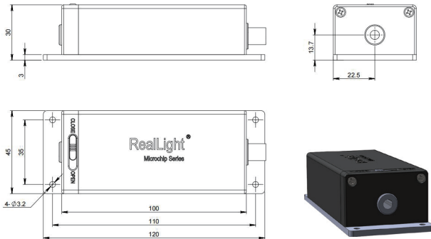
单脉宽激光头尺寸图
