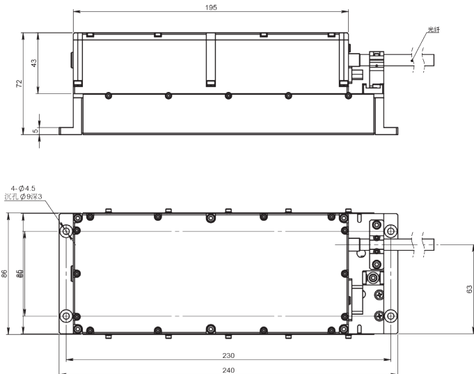
激光器尺寸
