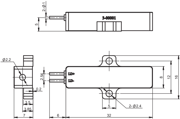
F3A尺寸图
