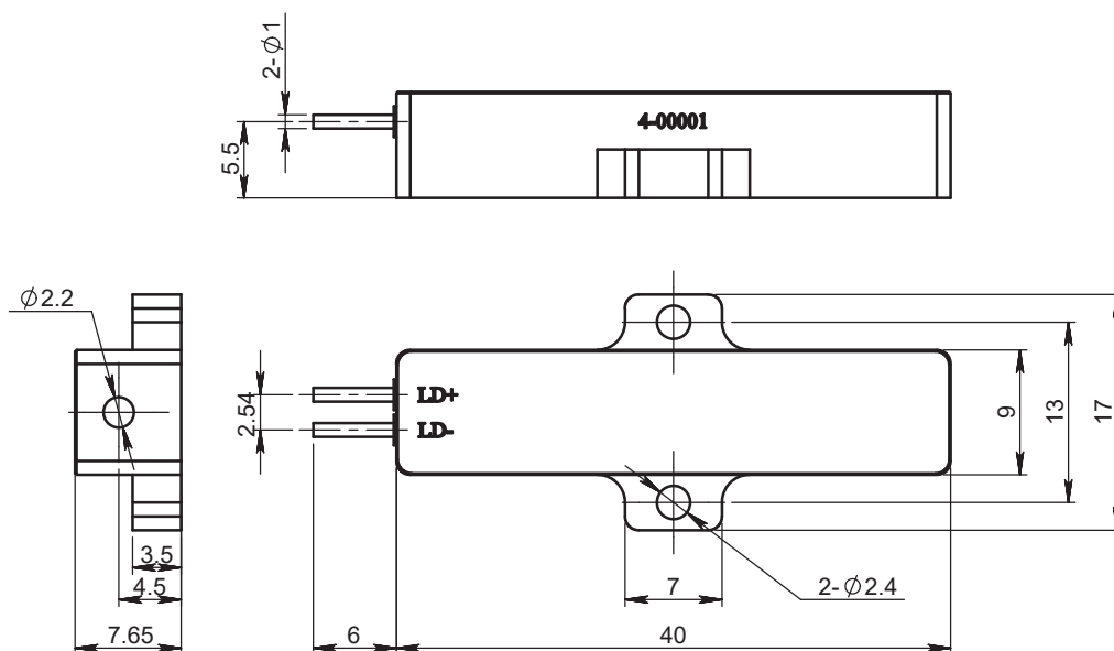
F4A尺寸图
