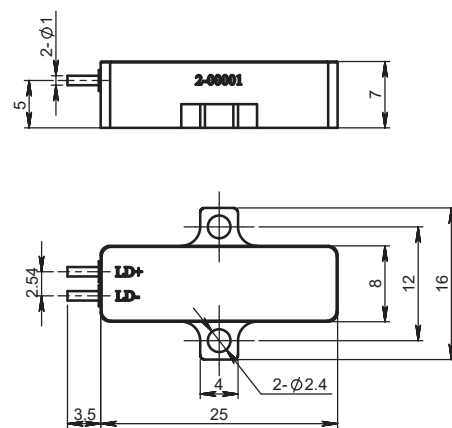
F2A尺寸图
