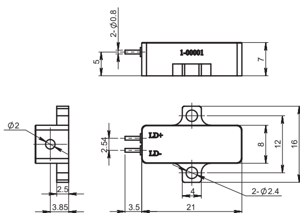
F1A尺寸图
