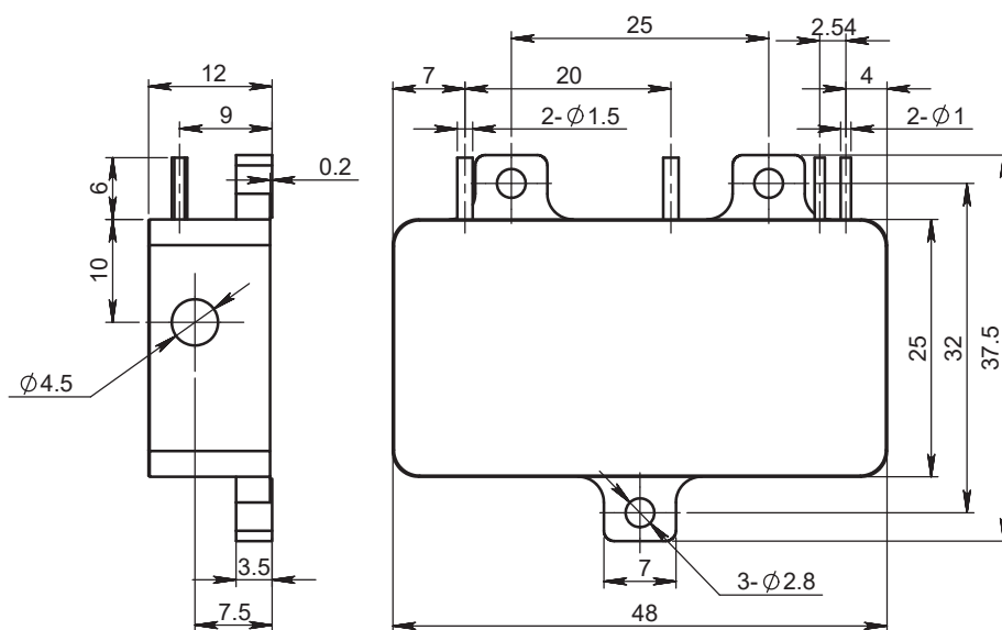
F11B尺寸图
