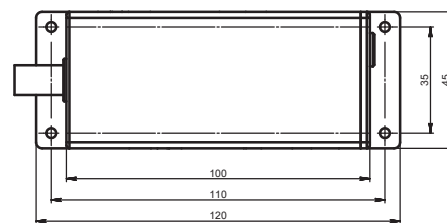
激光头尺寸图
