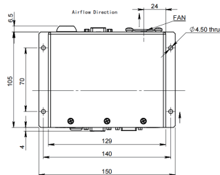
驱动电源尺寸图
