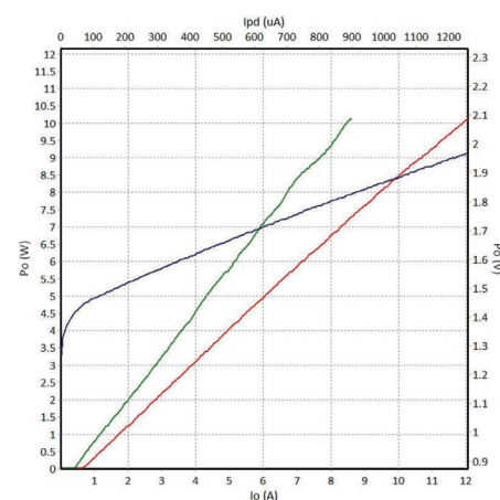
980nm P-I-V曲线图
