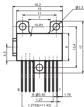
08LTR(L)-mini尺寸图
