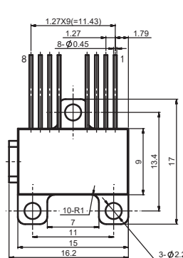
08LTR(R)-mini尺寸图
